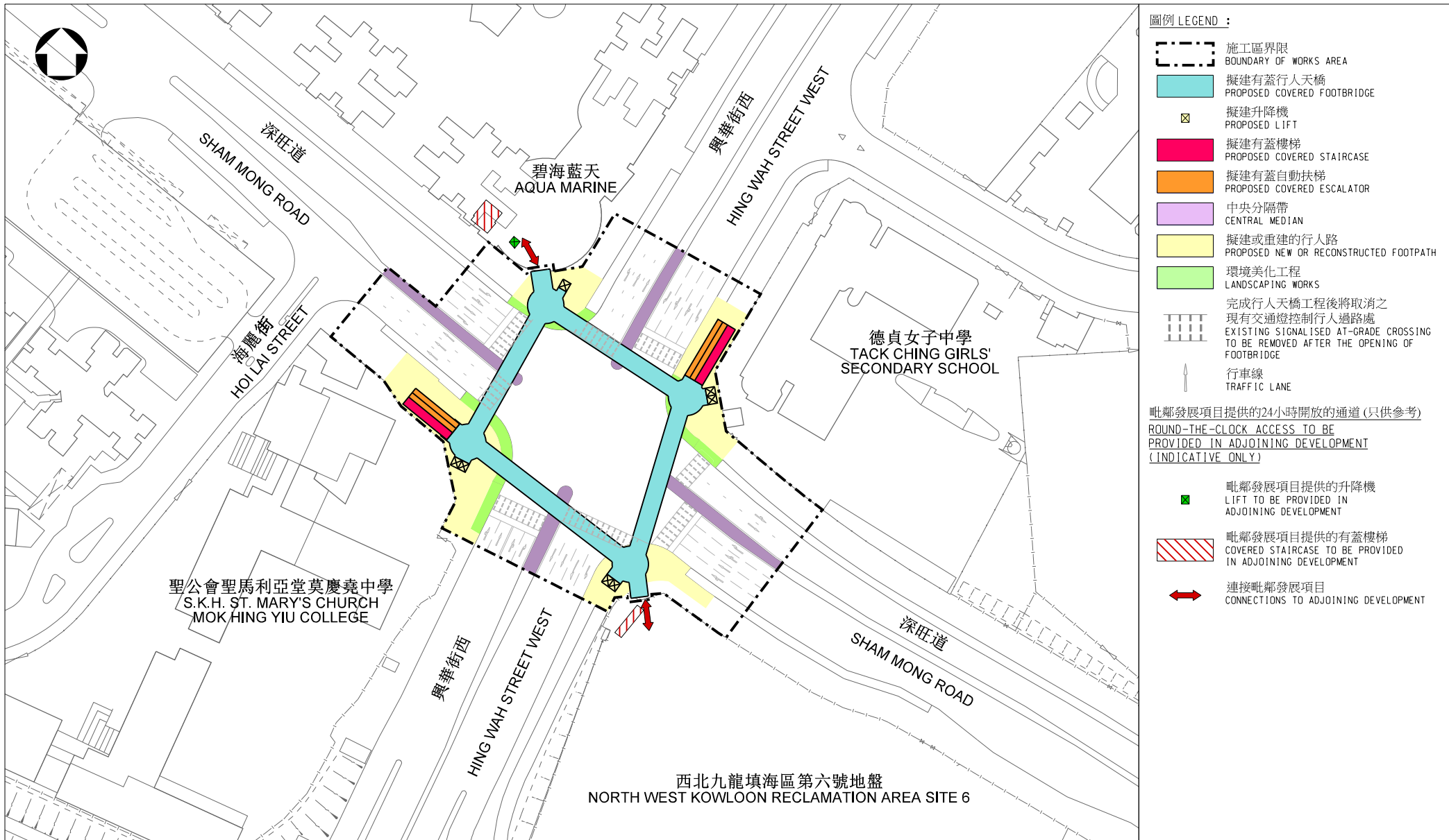
西九龍填海計劃 - 主要工程 (餘下部分) - 位於深水埗深旺道與興華街西交界處的行人天橋 - 平面圖
